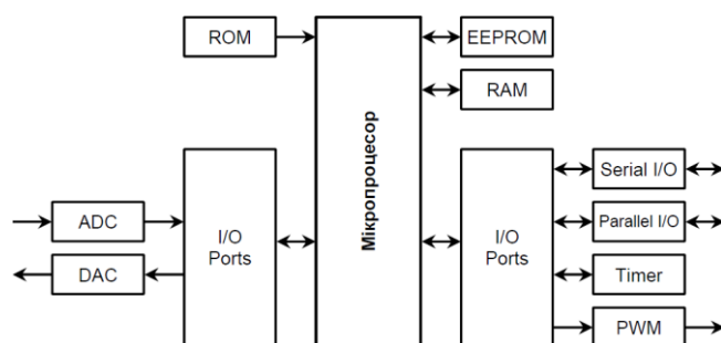
Рисунок 1.5 - Конфігурація мікропроцесора
