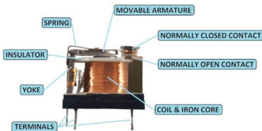
Рисунок 2.40 – Конструкція реле
