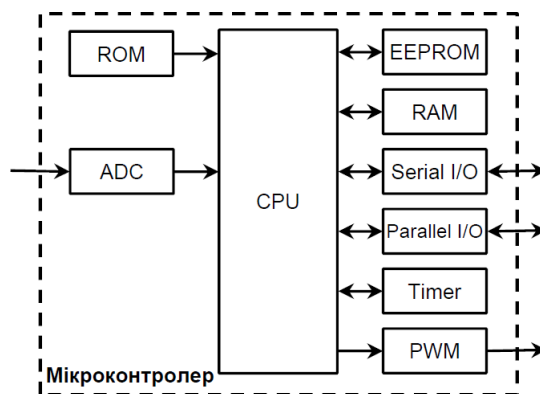
Рисунок 1.6 - Конфігурація мікроконтролера
