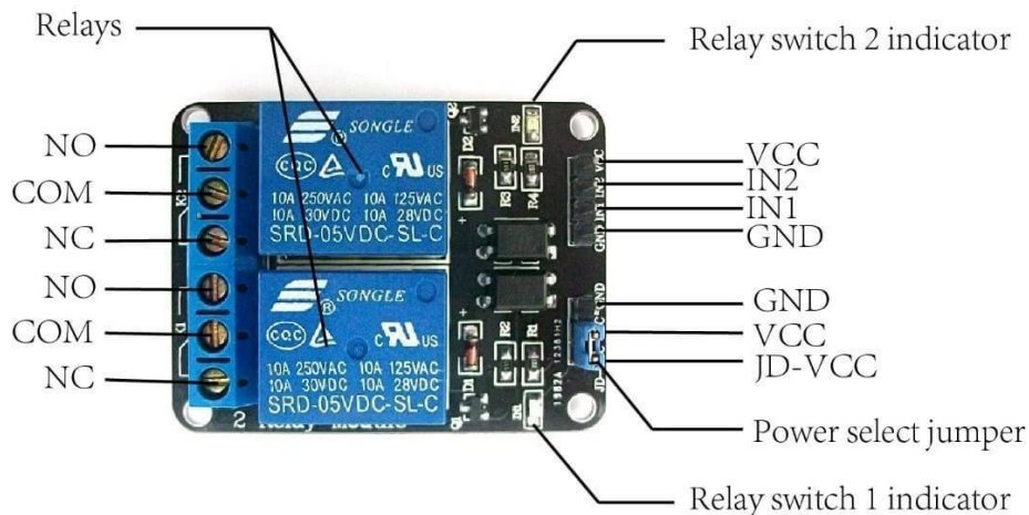
Рисунок 2.41 – 2х канальний реле модуль
